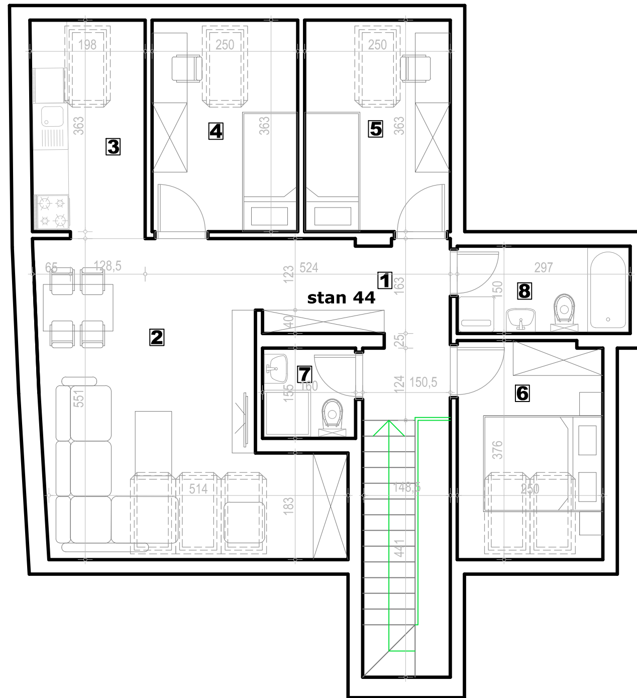
POTKROVLJE nivo II
